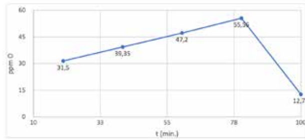
Şekil 9: Al cürufu ile deoksidasyon sonrasında 3. potadaki oksijen seviyesi değişimi
