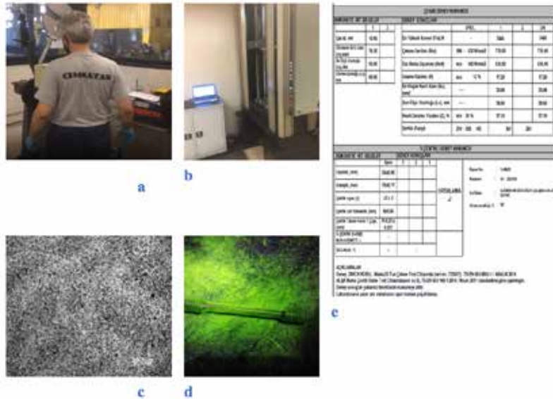
Şekil 10: a- Charpy Darbe Testi, b-Çekilme tet, c-mikroyapı, d-Floresan Manyetik Parçacık Muayenesi, e-Mekanik Test Sonuçları
