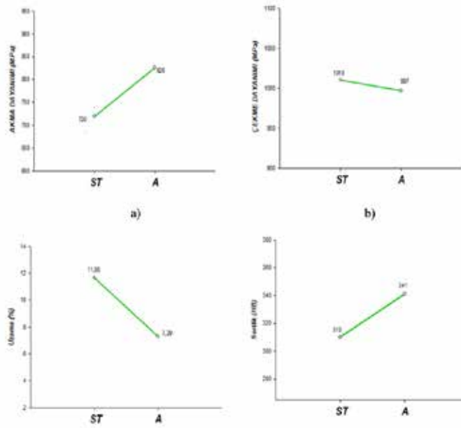
Şekil 2 : Östemperlenmiş numunelerin çekme ve sertlik değerleri a) Akma Dayanımı (MPa) b) Çekme Dayanımı (MPa) c) Uzama (%) d) Sertlik (HB) ST= Standart Numune, A=Bakırlı Numune
