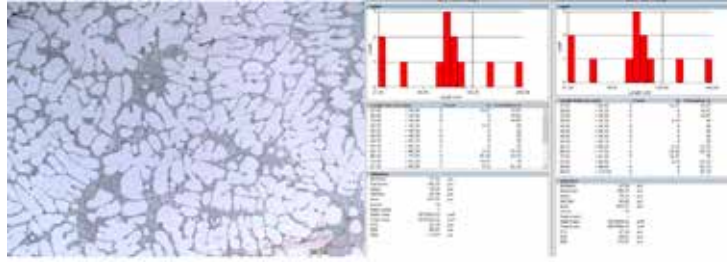
Şekil 9 : Döküm Sonrası SDAS Göbek 50x : ortalama = 76,3 \mu m
