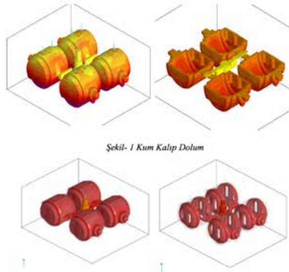
Şekil 2: Döküm Sonrası Katılaşma
