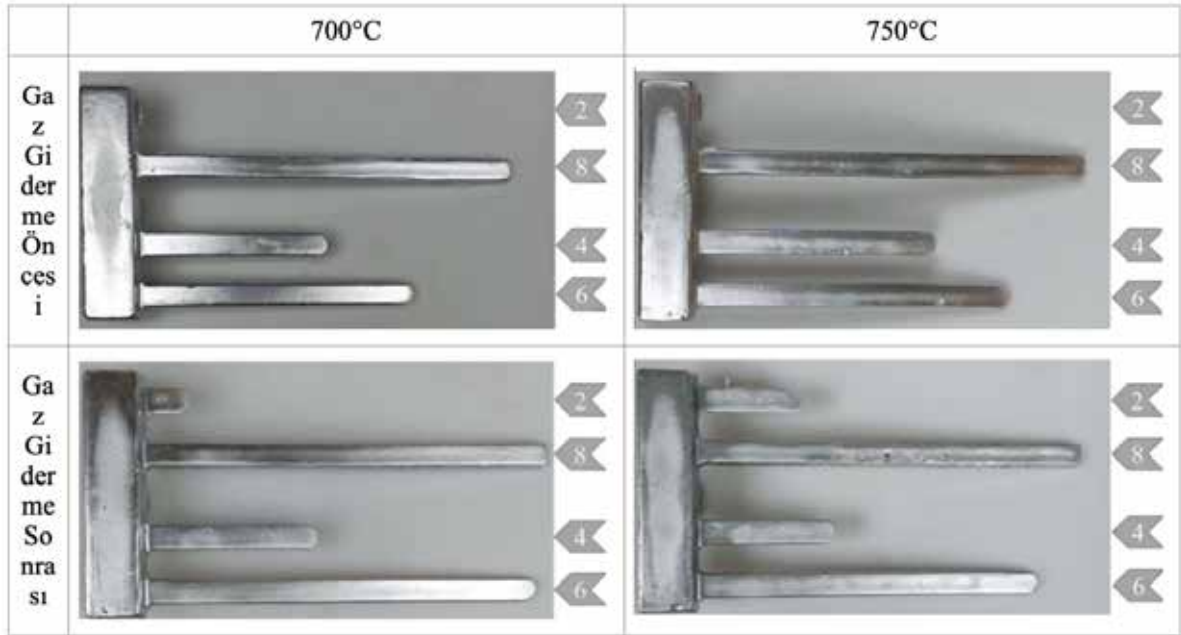
Şekil 3: 4 kanallı akıcılık numune fotoğraf görüntüleri
