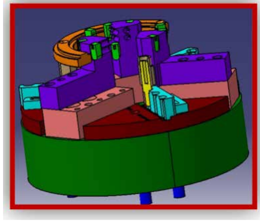
Resim 3: 10 nolu op. İçten dışı doğru ve aşağı doğru birlikte sıkma kesit görünüş
