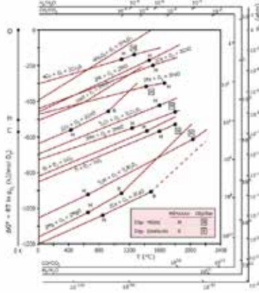
Şekil 1: Ellingham diyagramı
